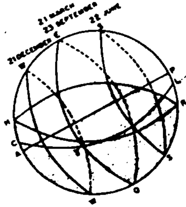
চিত্র-১ অয়ন ও বিষুব
