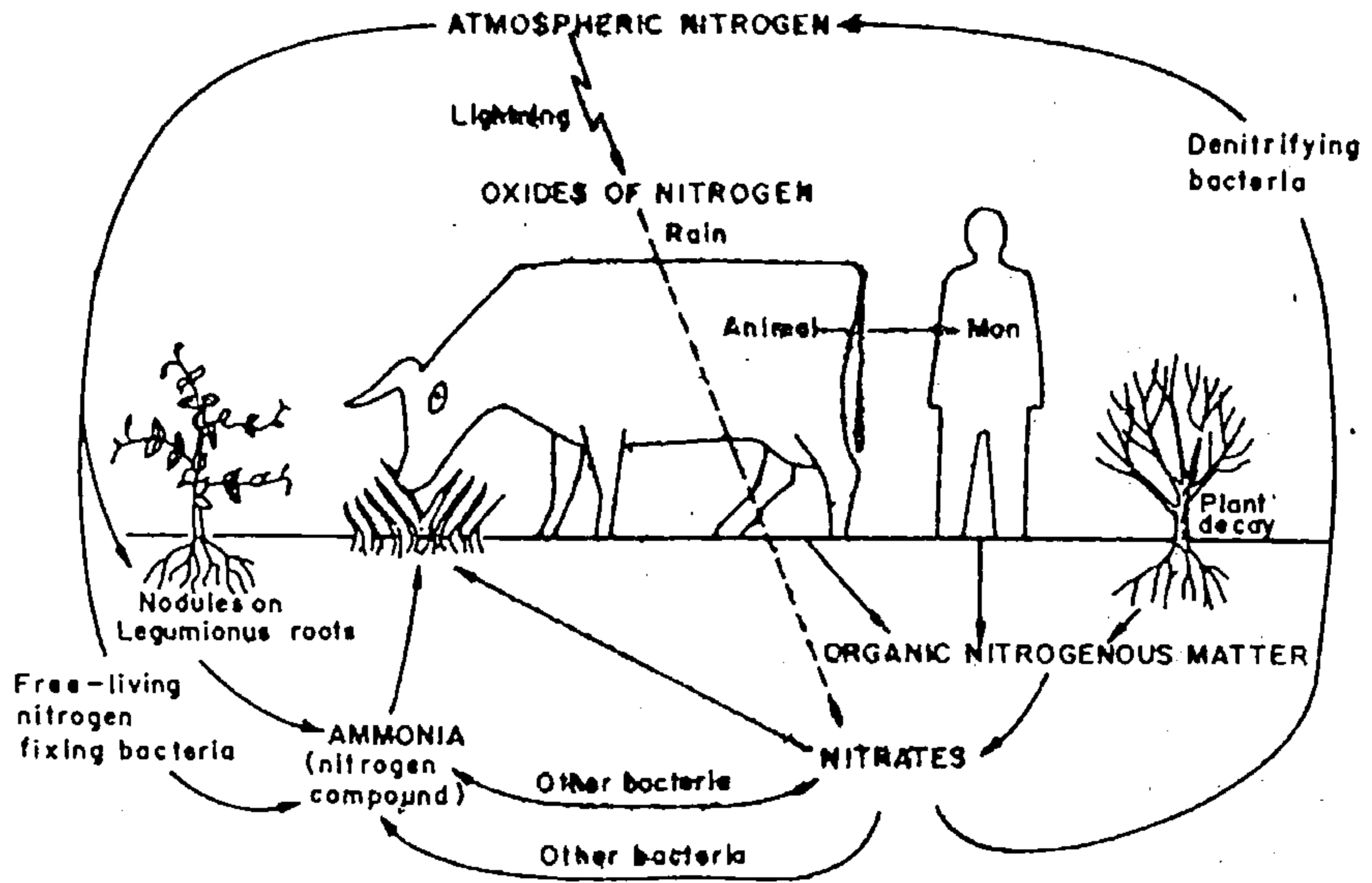
চিত্র- ৬ : নাইট্রোজেন চক্র
